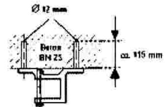
Bild 2b Deckenmontage
