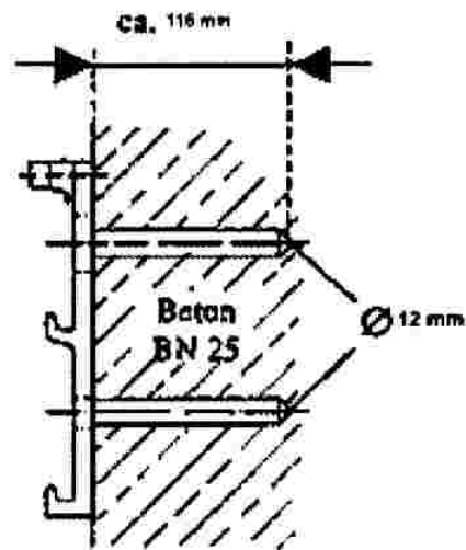
Bild 1b Wandmontage
